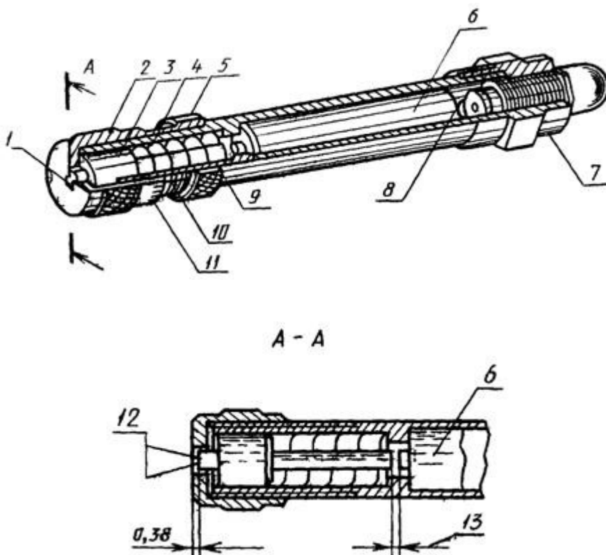
Устройство для определения остроты концов
