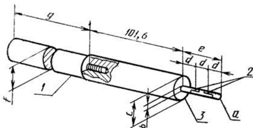
Зонд для проверки доступности
